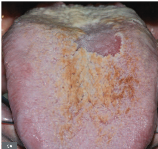
Fig. 3A. Glossite losangique paramédiane chez un homme fumeur et diabétique de type 2 non équilibré. B. Situation clinique 6 mois après prise en charge du diabète et traitement antifongique pendant 4 semaines (amphotéricine B), les papilles se sont reformées après plusieurs mois.
