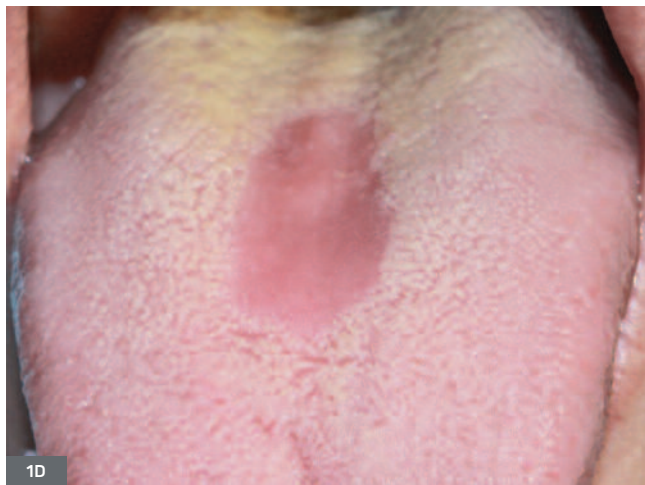
Fig. 1. Les différentes expressions cliniques de la glossite losangique médiane. D. Forme lisse d'aspect atrophique chez une femme en bonne santé générale et fumeuse. E. Forme lisse paramédiane chez un homme diabétique de type 2 non équilibré.
